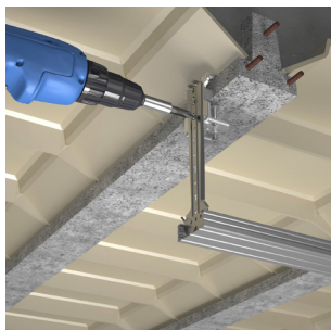
Fixation d'une suspente sur GRIP HM de PAI
