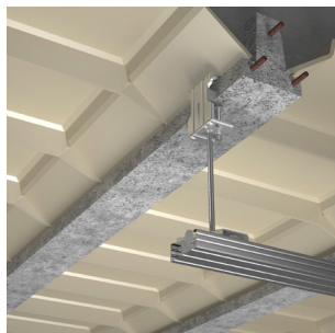
Vissage d'une tige filetée sur GRIP HM de PAI
