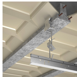
Accroche d'une suspente à réglage rapide sur GRIP HM de PAI
